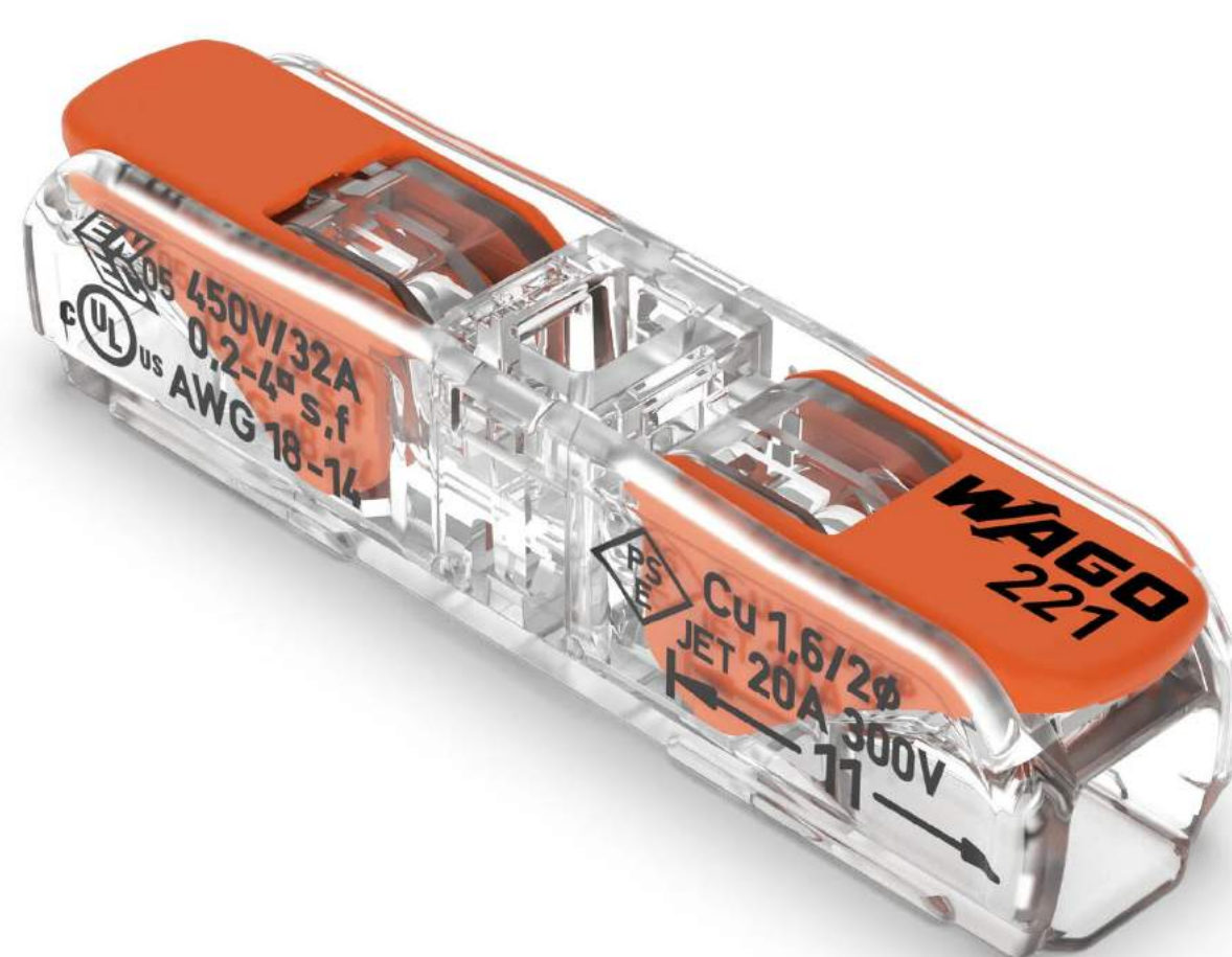
Клема пряма з нажимним важелем
